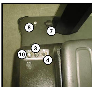
FIG.4 CONTROLS USED FOR STARTING WORK FIG.4 MANDOS PARA LA PRIMERA PUESTA EN FUNCIONAMIENTO DE LA BARREDORA FIG.4 COMMANDES POUR LA MISE EN SERVICE DE LA BALAYEUSE ABB.4 BEZUGSPUNKTE FÜR DIE ERSTE INBETRIEBNAHME DER KEHRMASCHINE FIG.4 PUNTI PER LA PRIMA MESSA IN FUNZIONE DELLA MOTOSCOPIA
