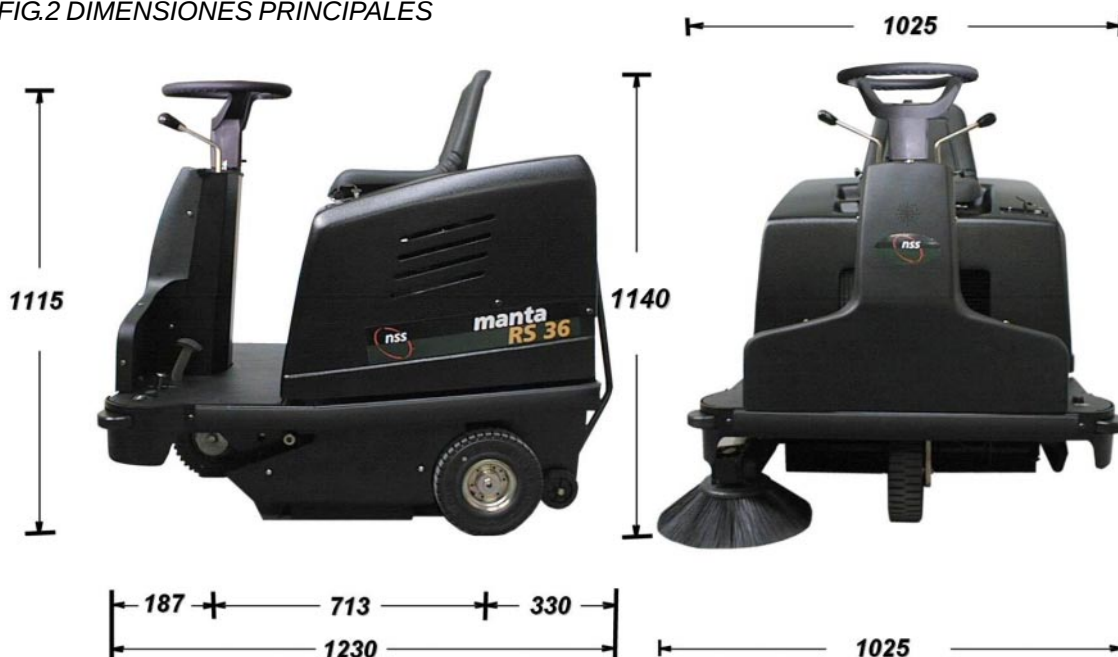
FIG.2 DIMENSIONES PRINCIPALES
