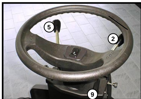
FIG.4 CONTROLS USED FOR STARTING WORK FIG.4 MANDOS PARA LA PRIMERA PUESTA EN FUNCIONAMIENTO DE LA BARREDORA FIG.4 COMMANDES POUR LA MISE EN SERVICE DE LA BALAYEUSE ABB.4 BEZUGSPUNKTE FÜR DIE ERSTE INBETRIEBNAHME DER KEHRMASCHINE FIG.4 PUNTI PER LA PRIMA MESSA IN FUNZIONE DELLA MOTOSCOPIA
