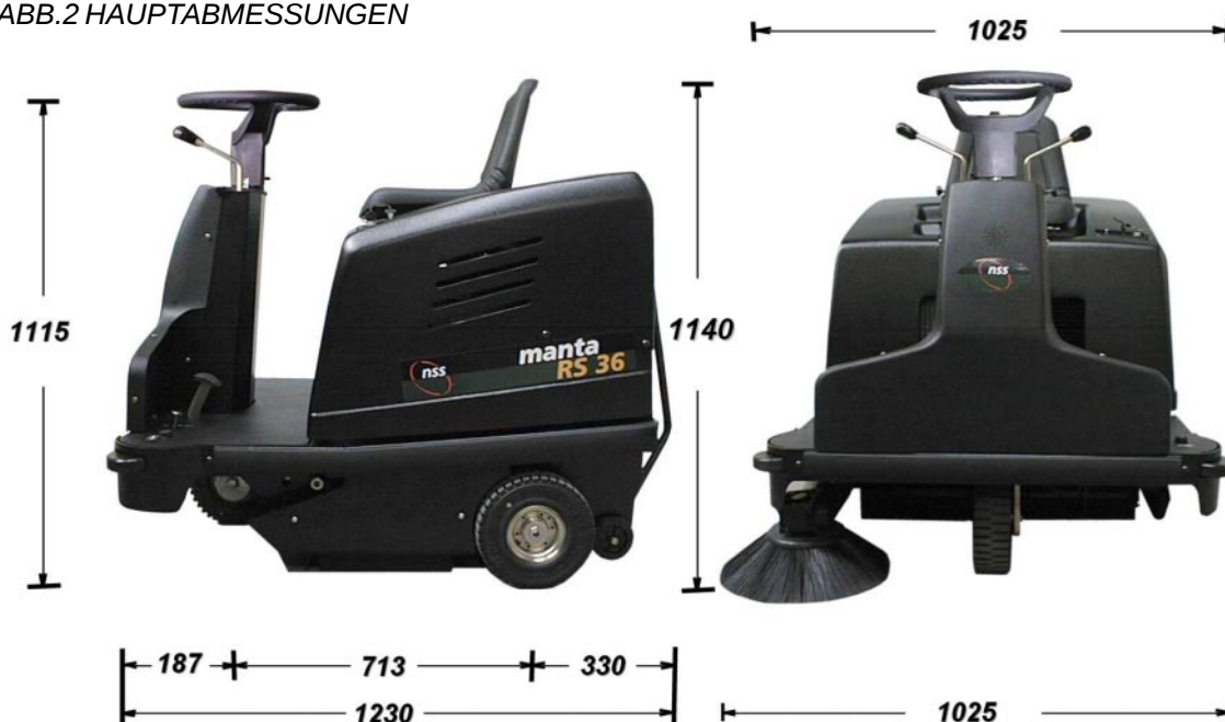
ABB.2 HAUPTABMESSUNGEN
