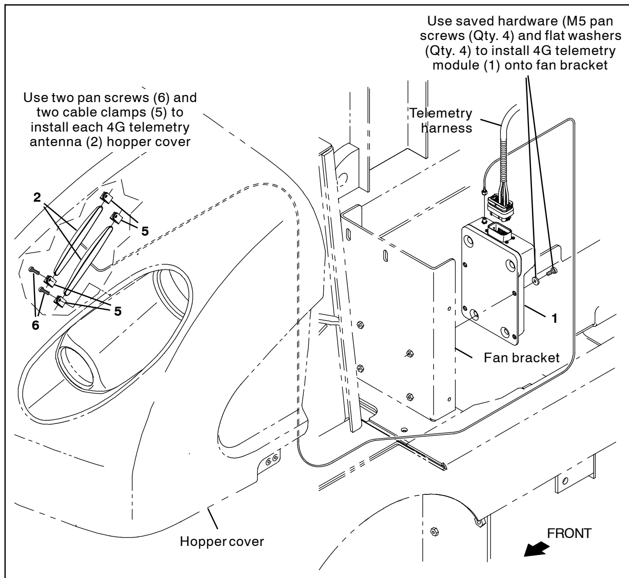
FIG. 11 - S30 Sweeper
