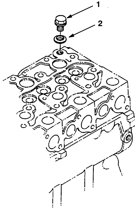
Fig. 22 - Plug
