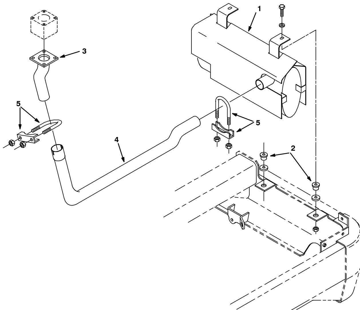
Fig. 23 - Muffler Group
