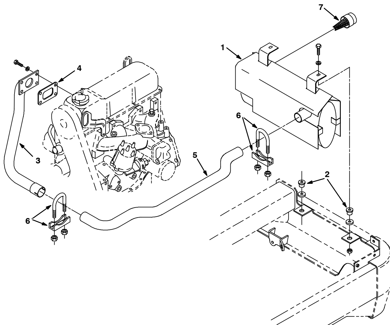
Fig. 26 - Muffler Group
