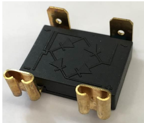
External rectifier
