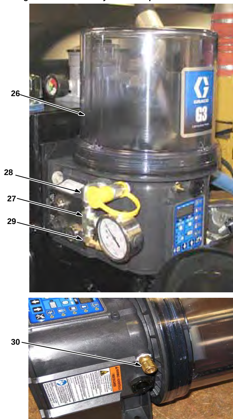
Fig. 41 – Auto-Lube System Group
