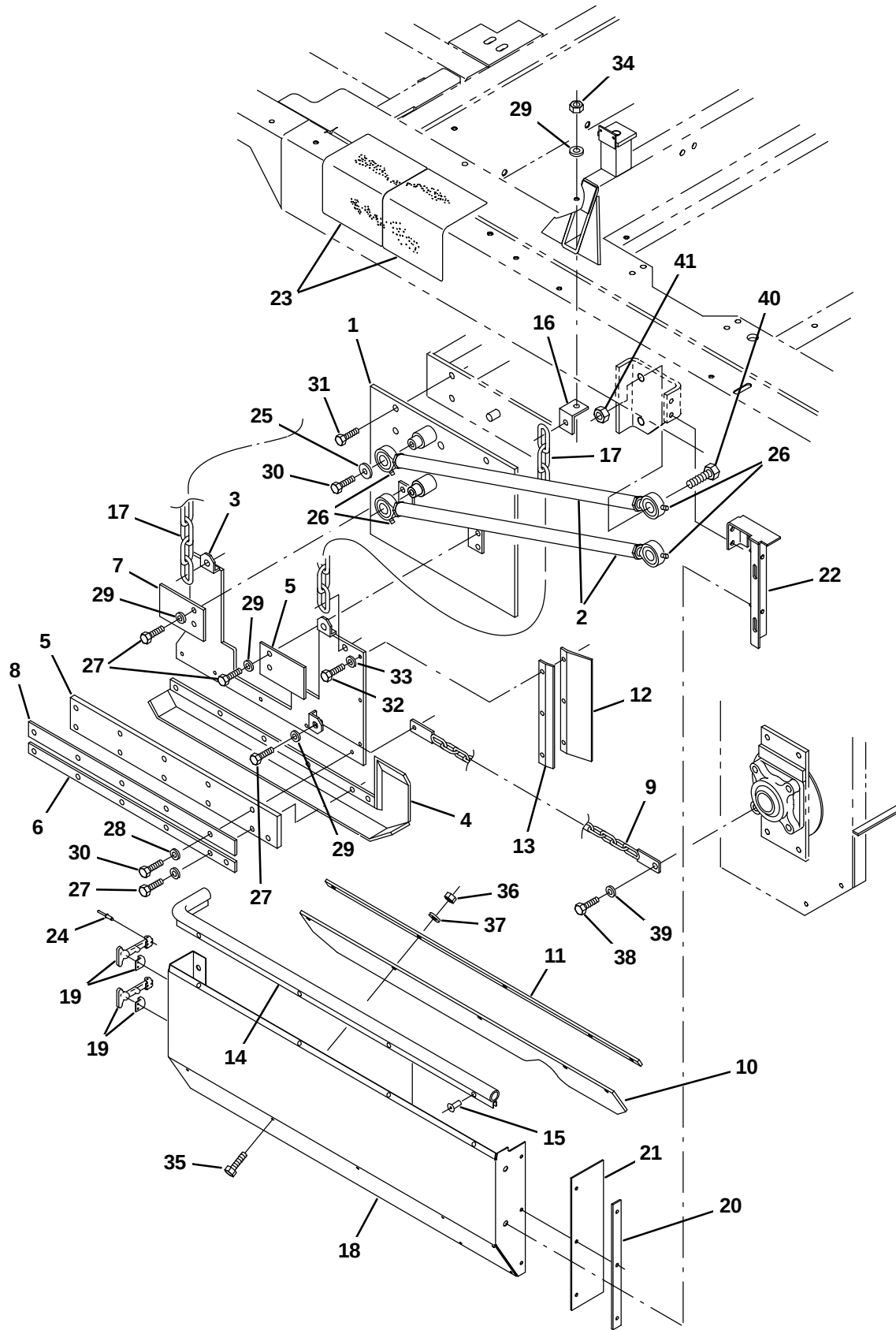
Fig. 5 – Main Frame, Right Brush Door Group
