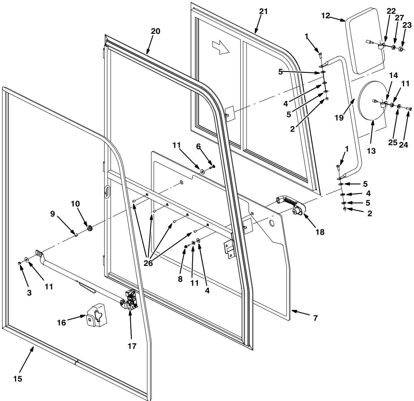
Fig. 45 – Cab Door Group, Left (S/N 009942– )
