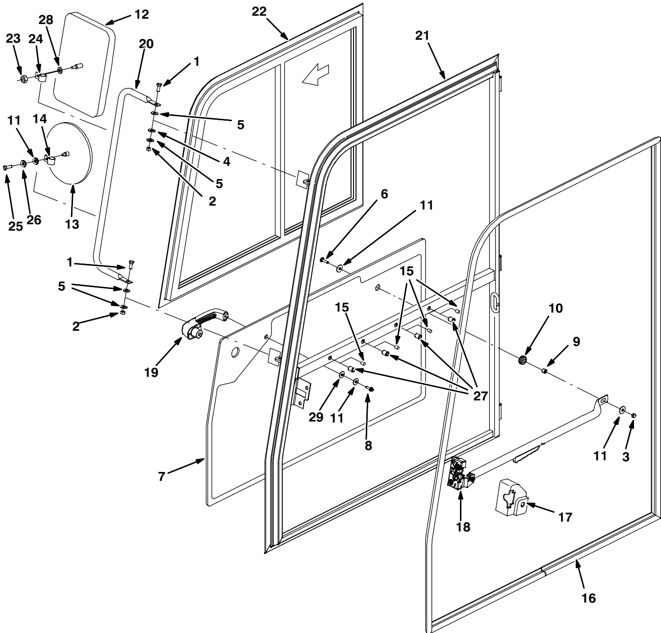
Fig. 43 – Cab Door Group, Right (S/N 009942– )
