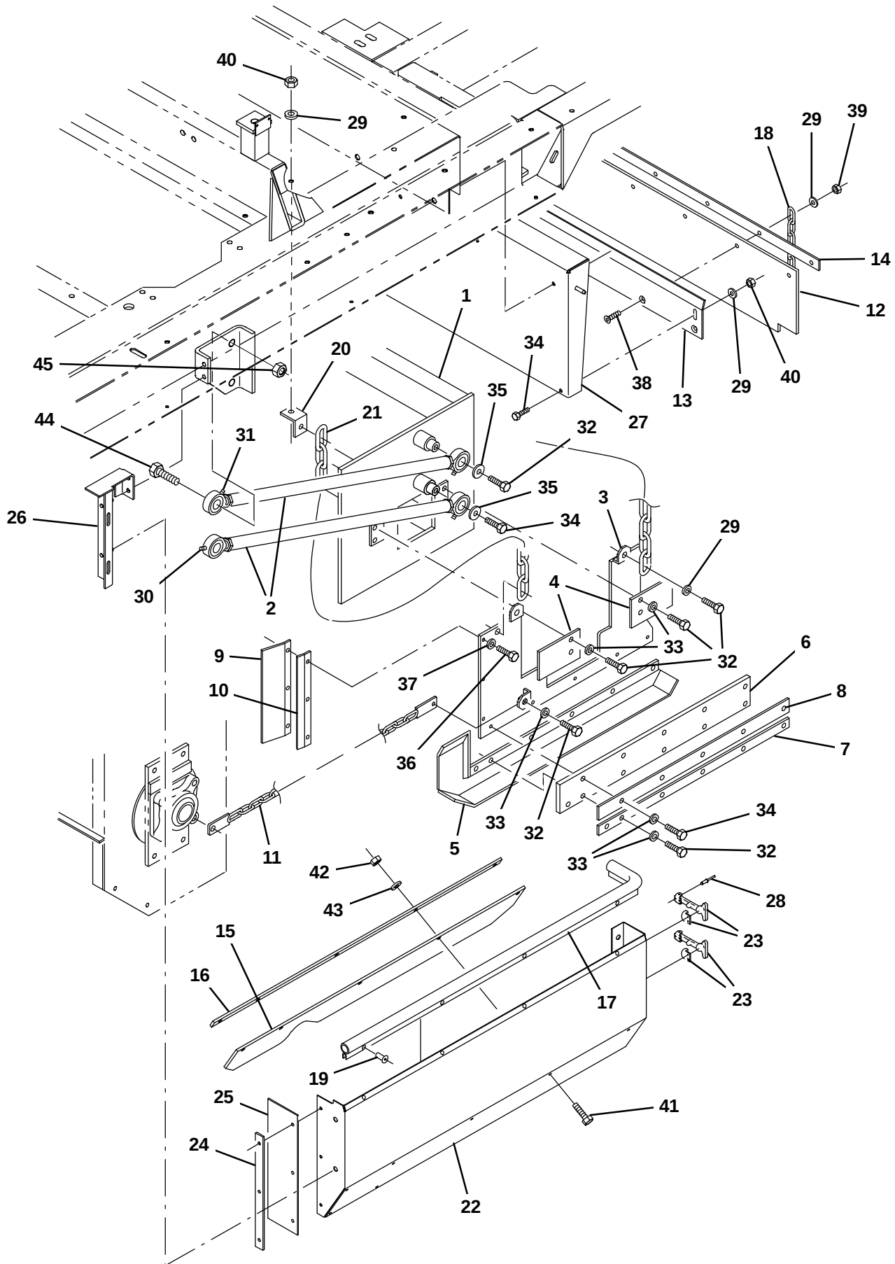
Fig. 6 – Main Frame, Left Brush Door Group
