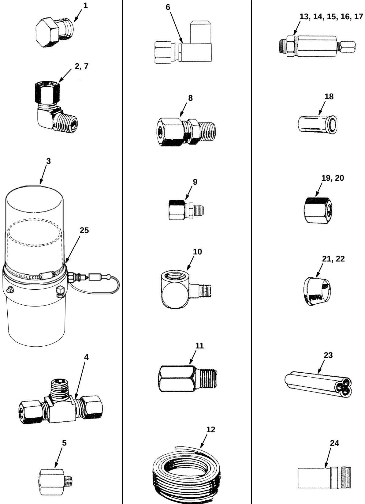
Fig. 41 – Auto-Lube System Group
