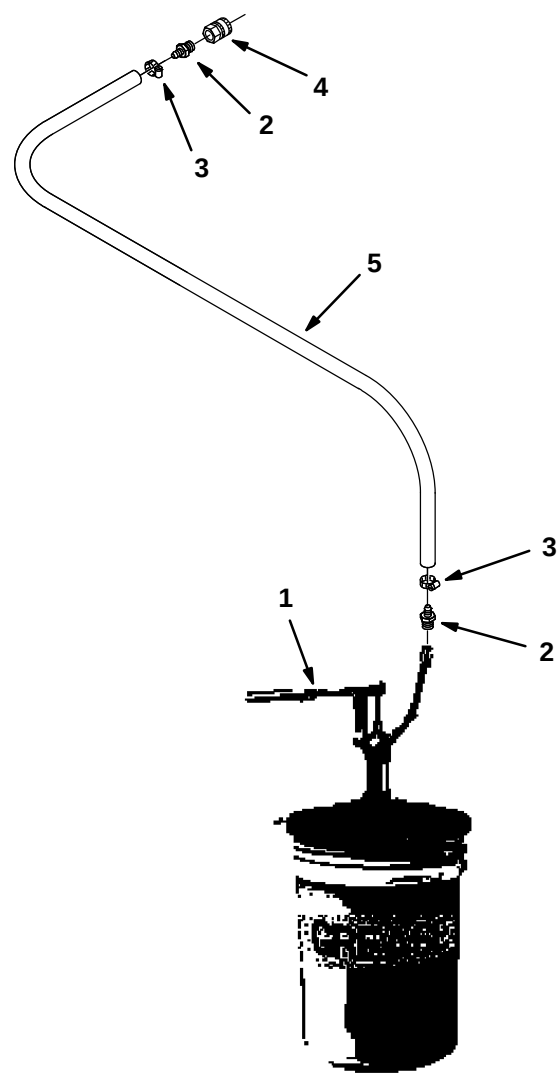
Fig. 42 – Auto-Lube Pump Kit
